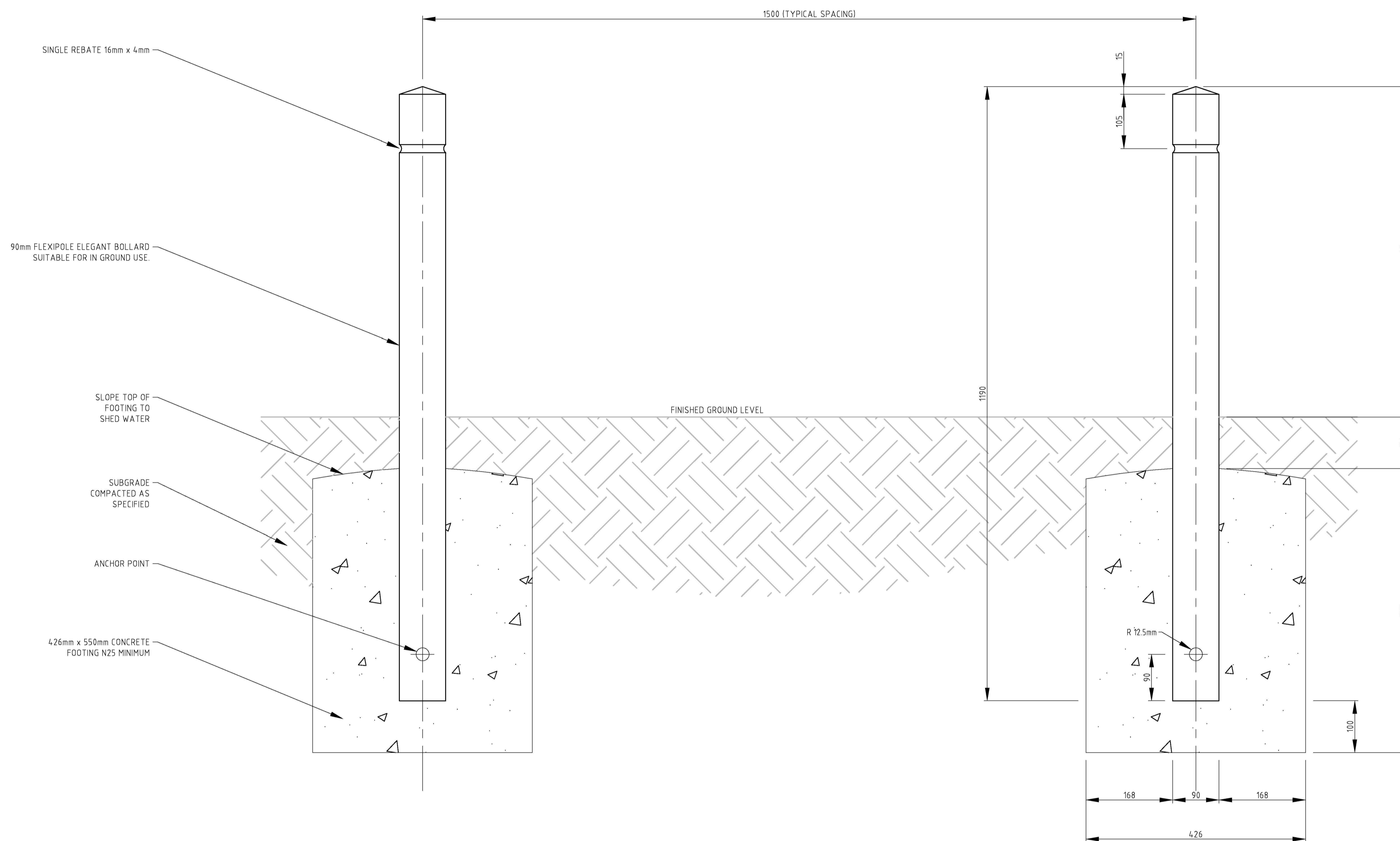
FLEXIPOLE ELEGANT FIXED BOLLARD N.T.S.
